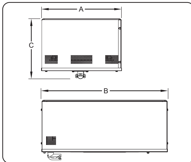
Dimensions — Modèles HWBIB-FUL (isolés, montage en bas)
