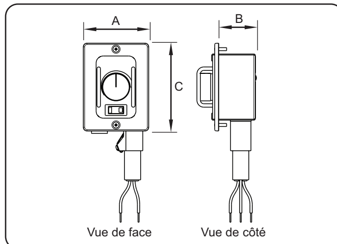
Dimensions du boîtier de commande
