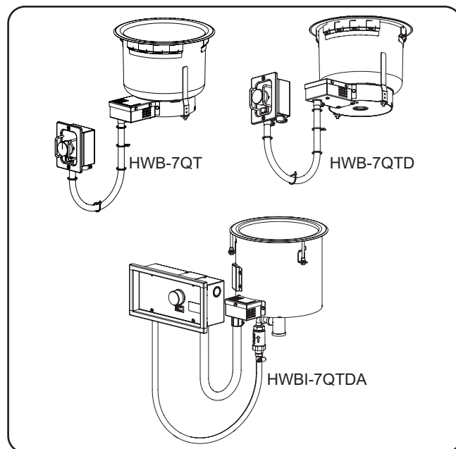
Modèles HWB-7QT et HWB-7QTD
