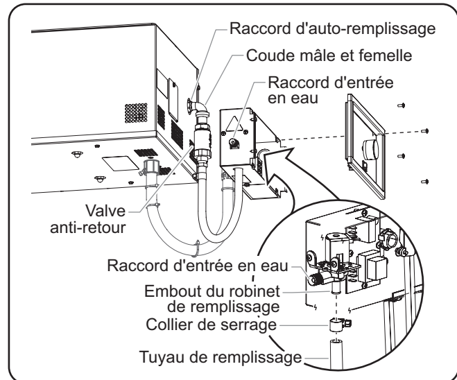
Installation de l'unité d'auto-remplissage (HWBIB-FULDA)
