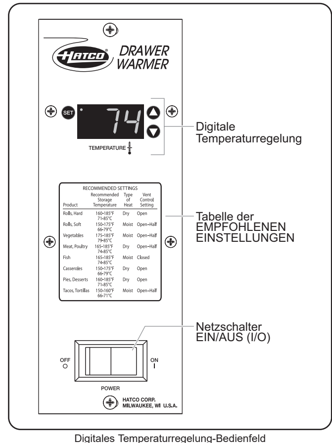
Digitales Temperaturregelung-Bedienfeld
