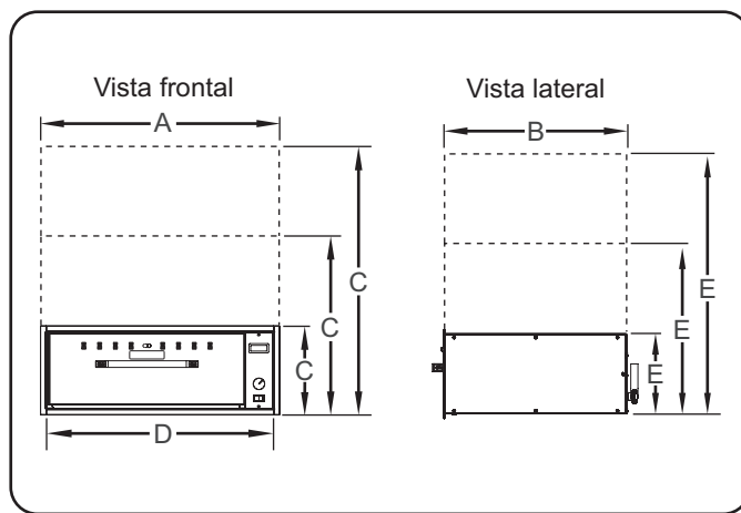
HDW-xB, HDW-xBN, y HDW-xBR Dimensiones
