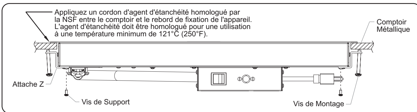
Modèle GRSBF — Installation
