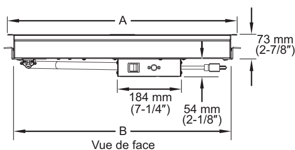
Dimensions — Modèles GRSB
