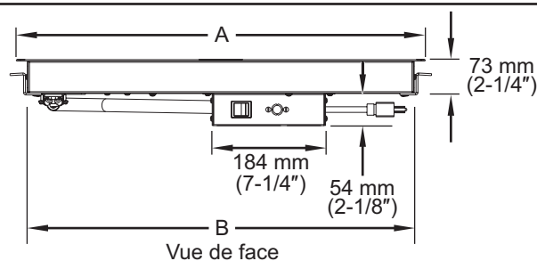
Dimensions — Modèles GRSBF
