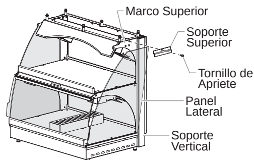
Instalación de un panel lateral
