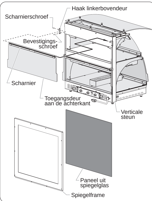
De toegangsdeuren aan de achterkant plaatsen
