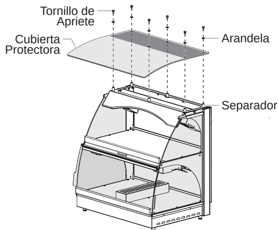
Instalación de la cubierta protectora
