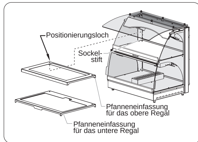
Pfanneneinfassungen
