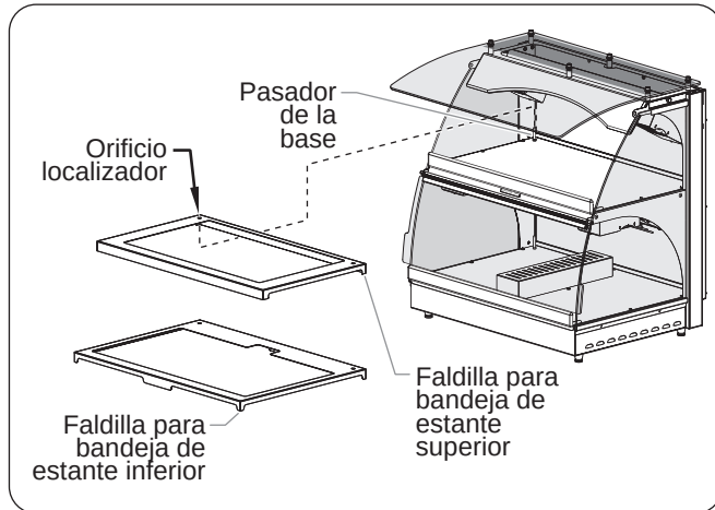
Instalación de las faldillas para bandejas
