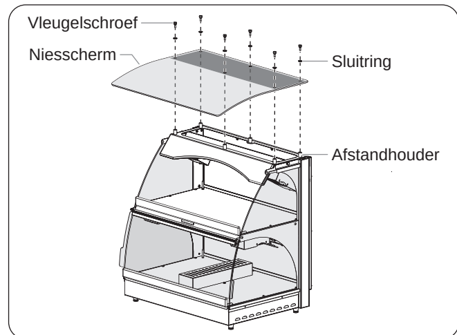
Het niesschermscherm plaatsen
