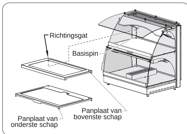
Panplaten
