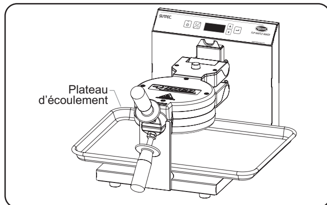
Installation du plateau d'écoulement
